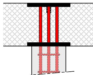
Plaque de tête et de reprise
