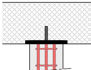
Plaque de tête avec goujon
