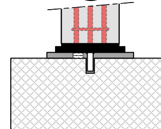
Pilier avec plaque de base sur dalle inférieure
