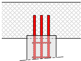
Armatures en attente
