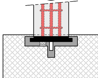
Pilier avec plaque de base dans engravure
