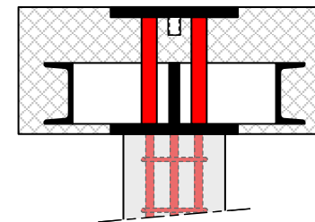
Tête anti-poinçonnement et reprise
