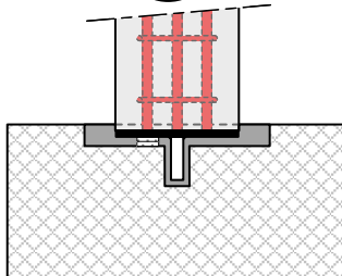
Pilier dans engravure
