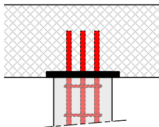
Plaque de tête avec armature
