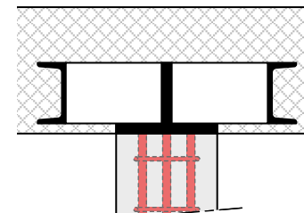
Tête anti-poinçonnement soudée
