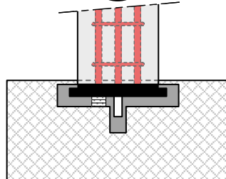
Colonne avec plaque de base dans engravure
