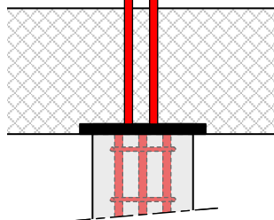
Plaque de tête avec armatures en attente
