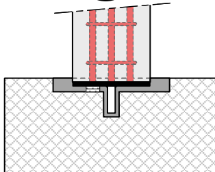
Colonne dans engravure
