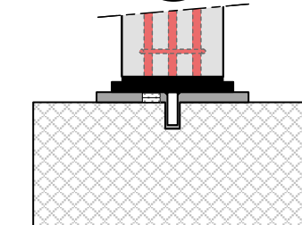
Colonne avec plaque de base sur dalle inférieure
