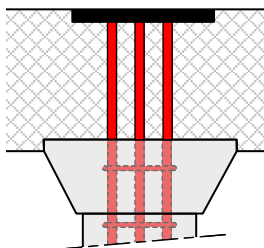
Champignon béton
