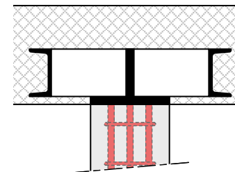
Tête anti-poinçonnement soudée
