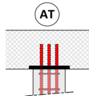
Plaque de tête avec armature
