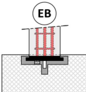
Colonne avec plaque de base dans engravure
