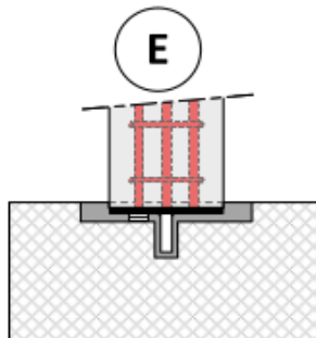
Colonne dans engravure
