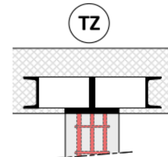
Tête anti-poinçonnement soudée
