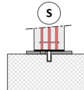
Colonne sur dalle inférieure
